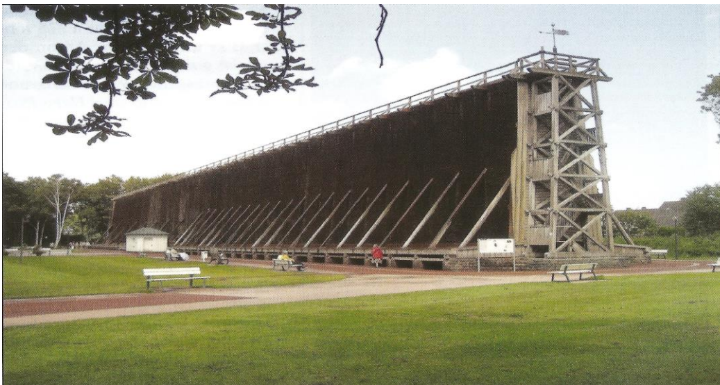
Abb. 4: Das 1835 nach Plänen von Pfarrer Philipp Korte erbaute Gradierwerk I im Kurpark von Bad Westernkotten [zitiert nach dem Aufsatz von Kennemann]
